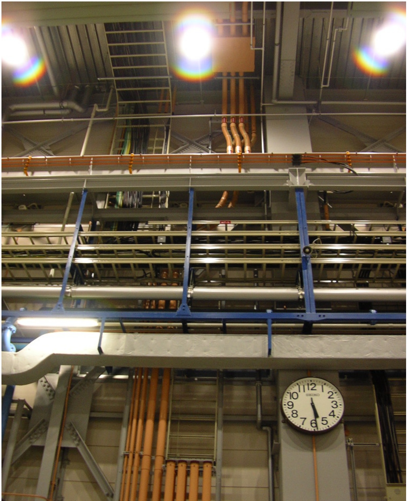
高圧幹線ケーブル布設工事(高さ18m) (株)ダイダン 日阪製作所(東大阪)6KV-CVT-150
